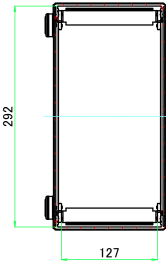
B-B ( 1 : 5 )
