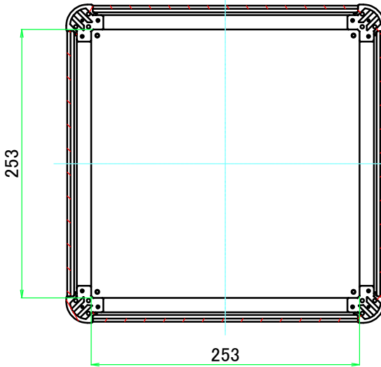
C-C ( 1 : 5 )
