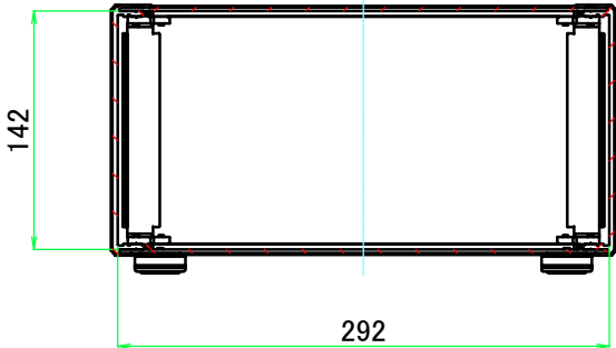
A-A ( 1 : 5 )
